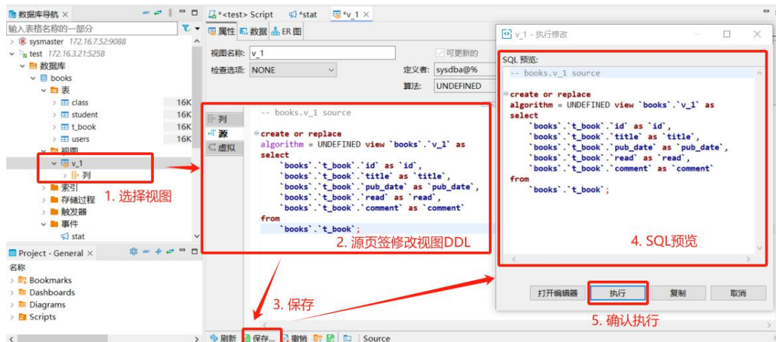
图 3-21 编辑视图
