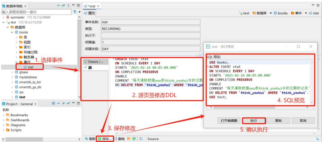
图 3-44 编辑事件
