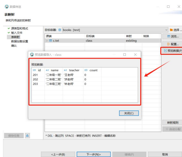
图 3-61 数据预览
