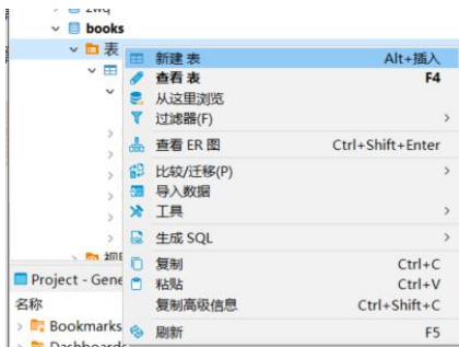
图 3-10 新建表
