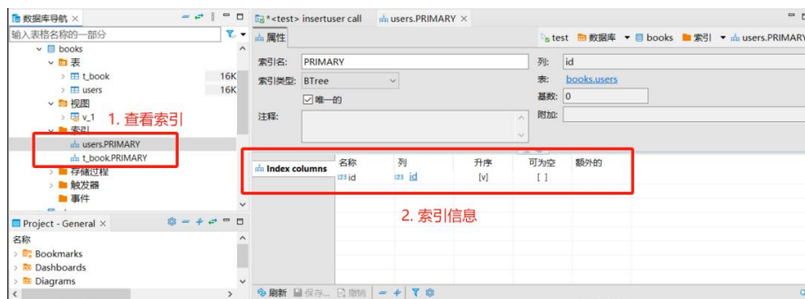
图 3-24 查看索引
