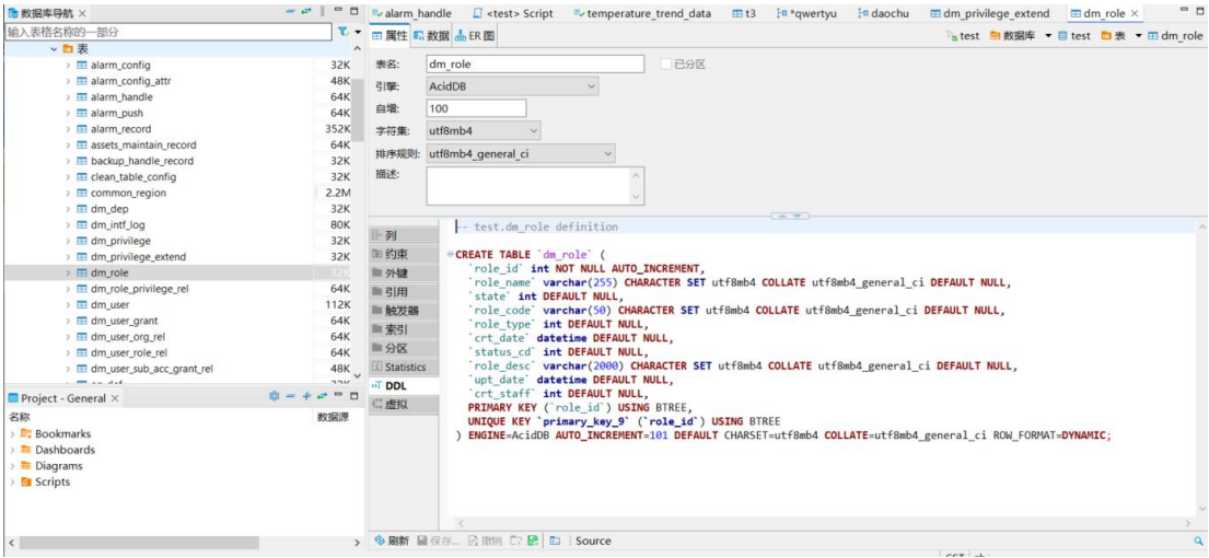
图 3-13 查看表属性
