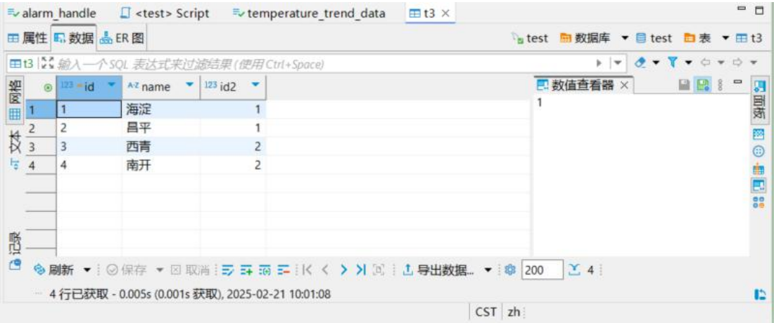
图 3-15 管理表数据
