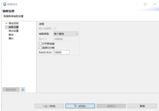
图 3-51 抽取设置
