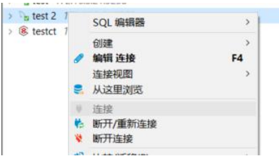
图 2-7 断开连接
