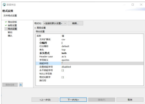
图 3-52 格式设置
