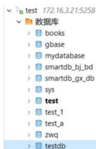
图 3-3 数据库列表
