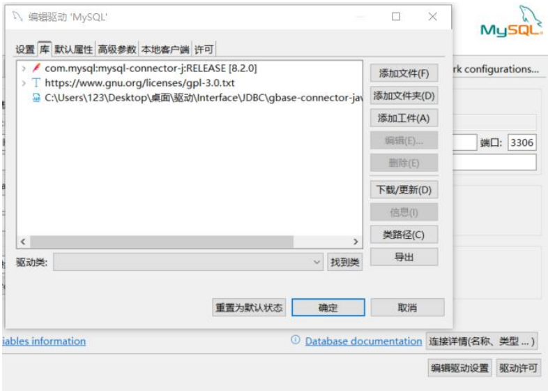
图 2-4 上传驱动
