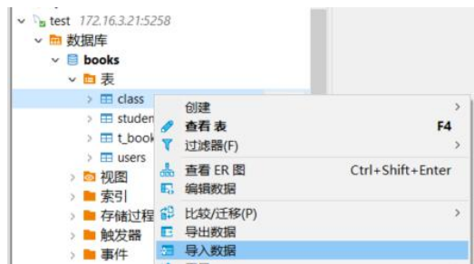
图 3-57 导入数据
