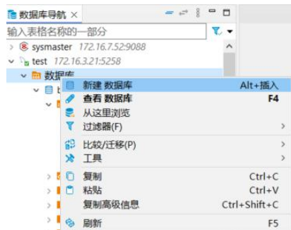
图 3-1 新建数据库
