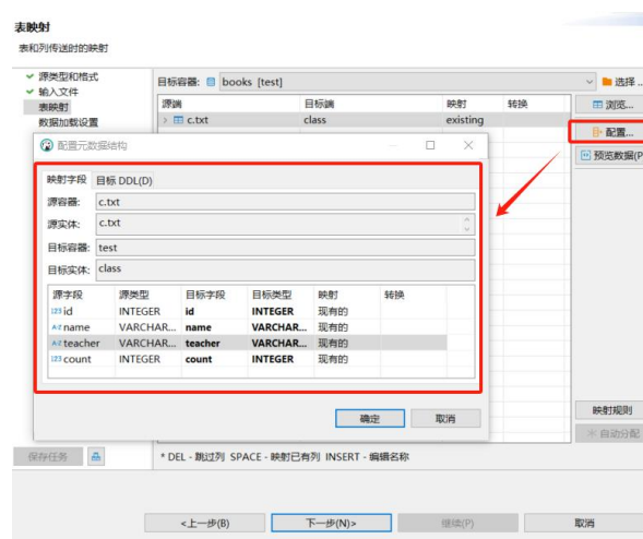
图 3-60 字段映射
