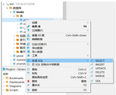
图 3-48 生成SQL
