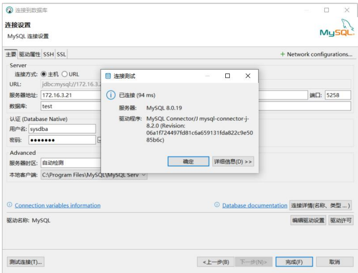
图 2-5 测试连接
