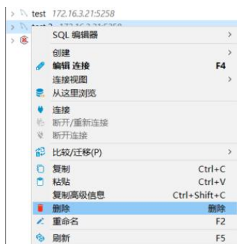
图 2-10 删除连接
