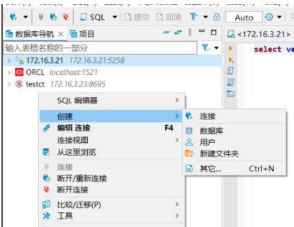
图 2-1 创建连接
