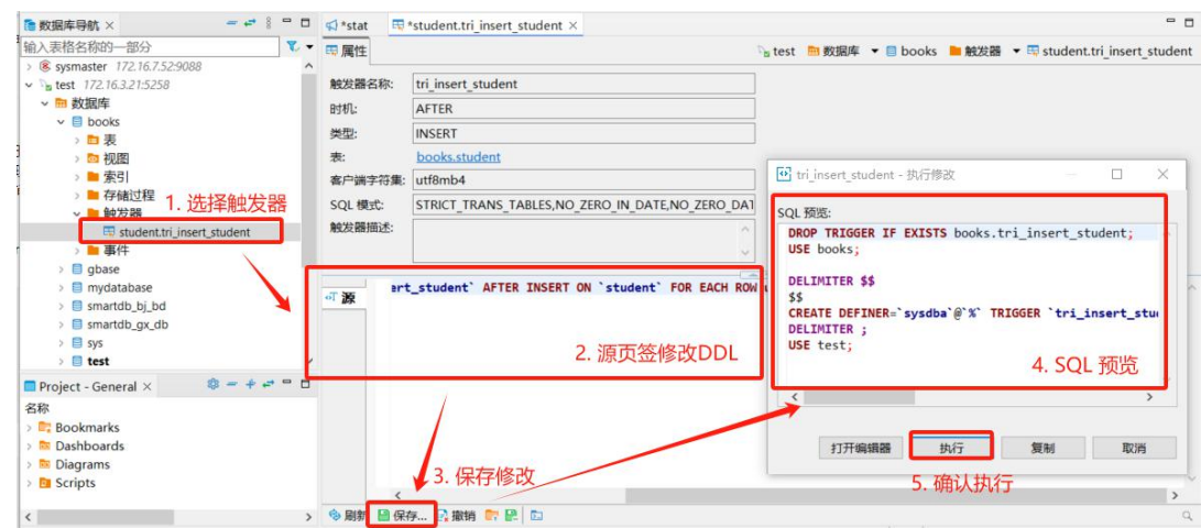
图 3-37 编辑触发器
