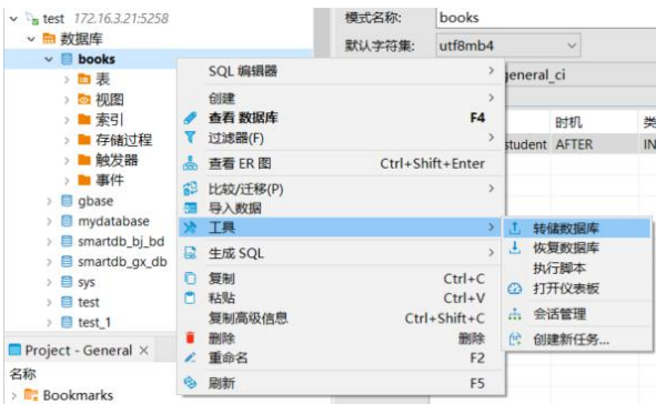
图 3-6 转储数据库
