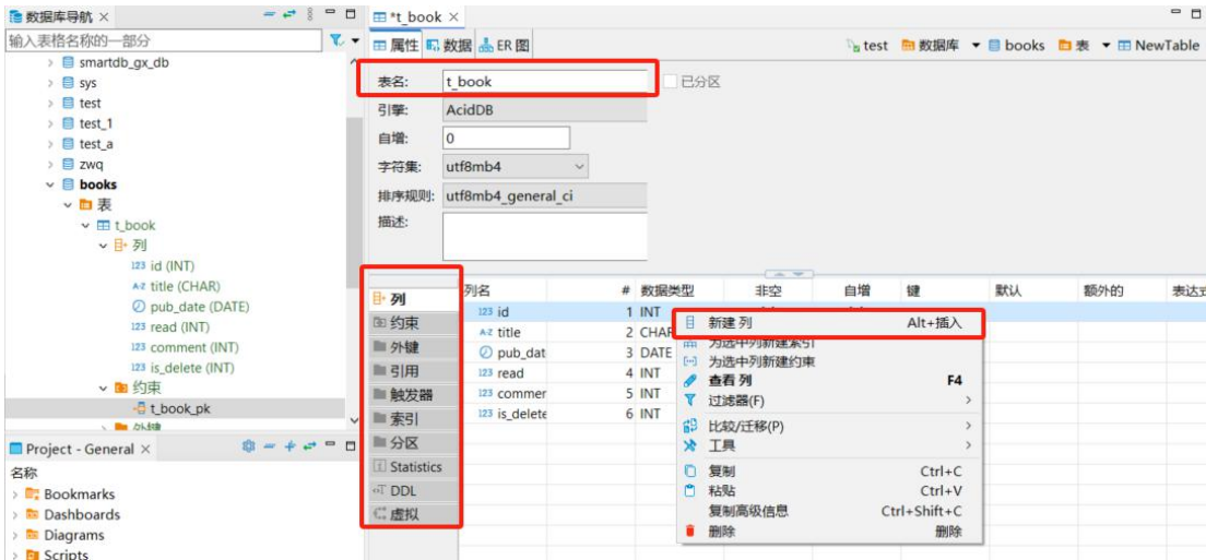
图 3-11 输入表信息
