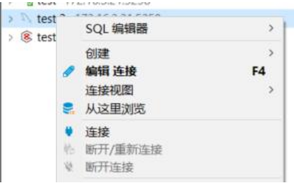
图 2-6 打开连接
