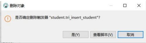
图 3-38 删除触发器
