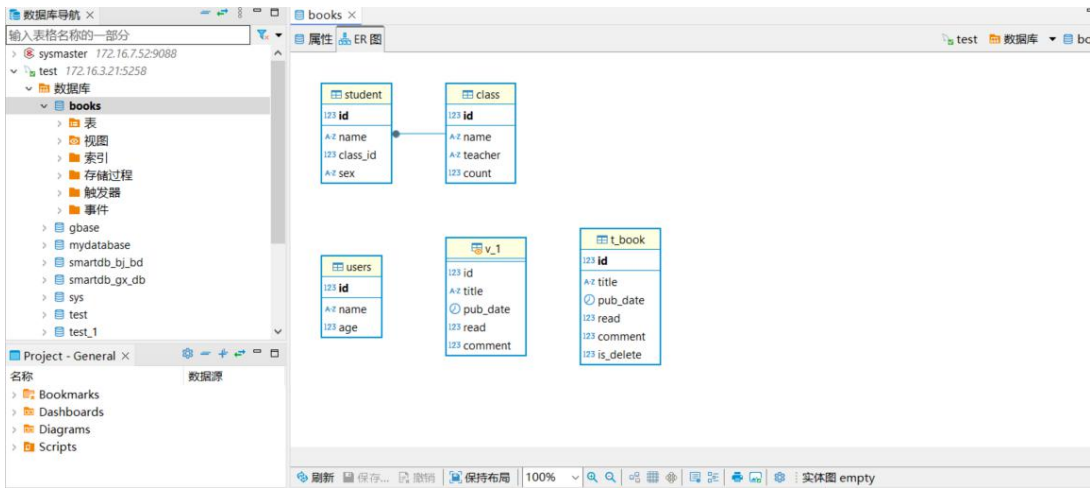
图 3-5 查看ER图
