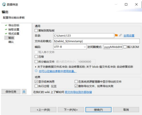
图 3-53 输出设置
