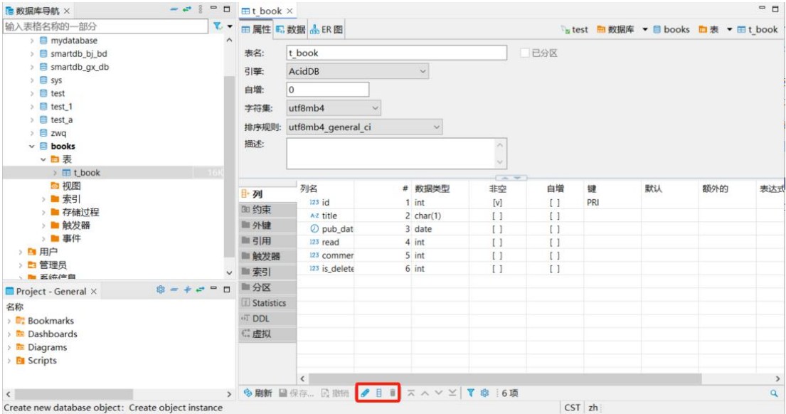
图 3-14 编辑表
