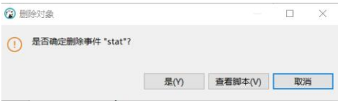
图 3-45 删除事件
